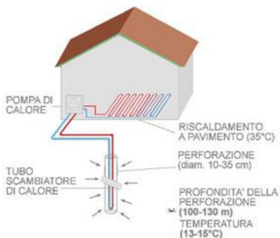
Schema di funzionamento di un impianto geotermico con pompa di calore e impianto di riscaldamento radiante
